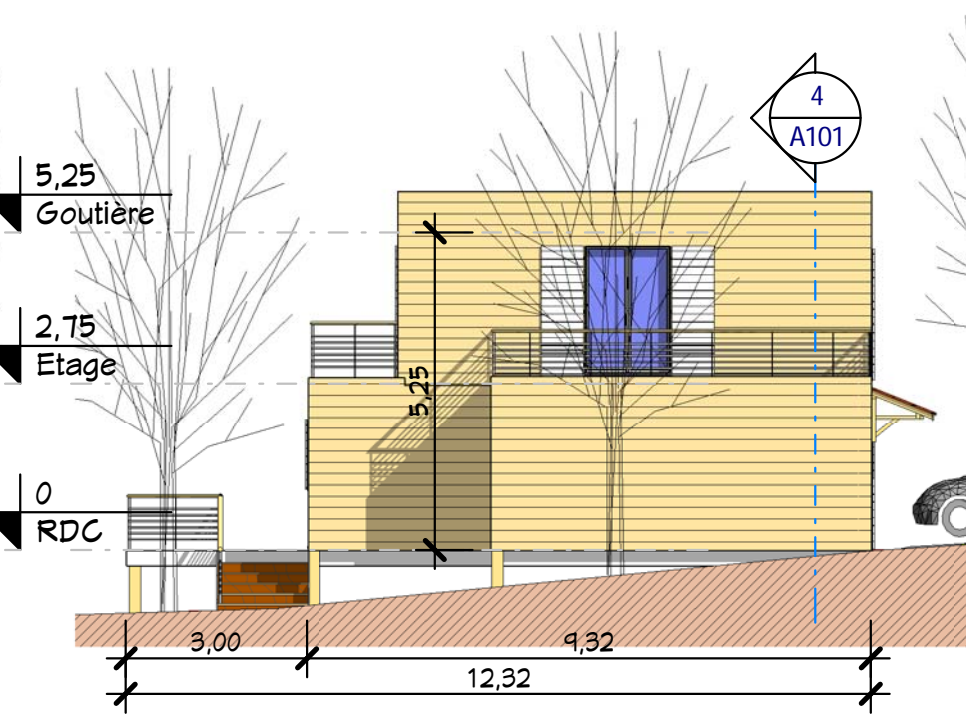
4 Elév. Sud Ech : 1 : 125
