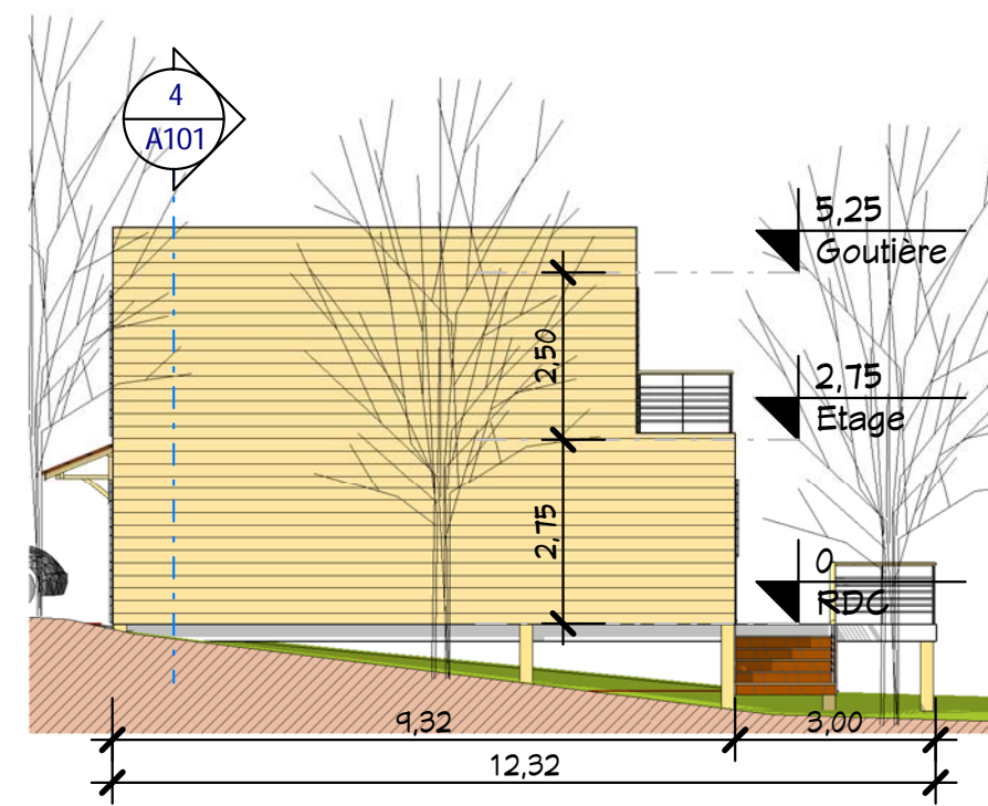
5 Elév. Nord Ech : 1 : 125
