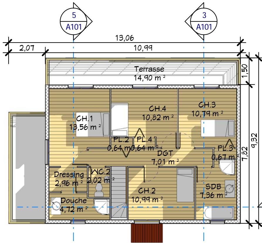
2 Etage Ech : 1 : 125
