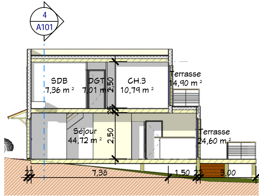
3 Coupe 1 Ech : 1 : 125
