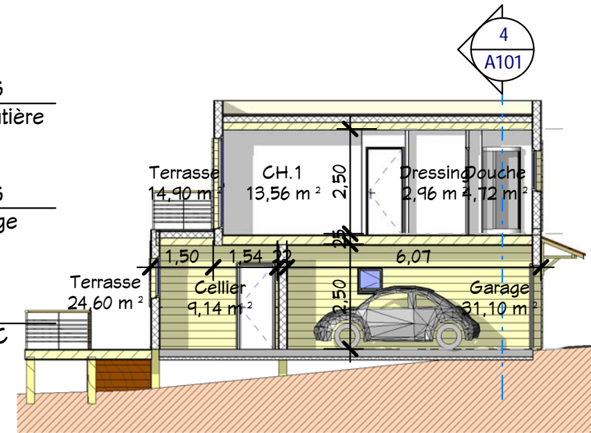
5 Coupe 3 Ech : 1 : 125
