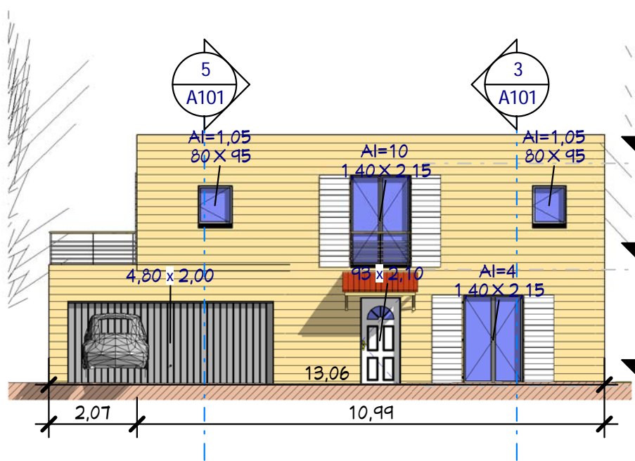
2 Elév. Est Ech : 1 : 125
