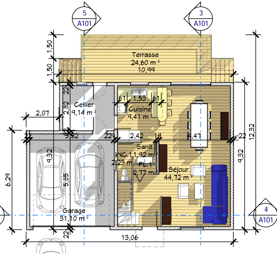
1 RDC Ech : 1 : 125
