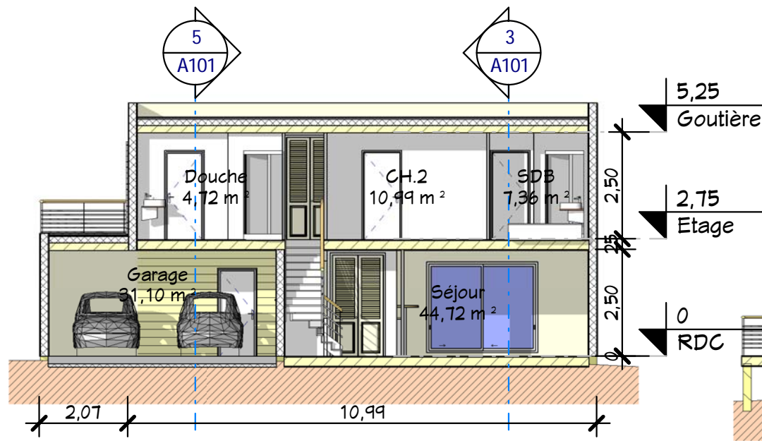
4 Coupe 2 Ech : 1 : 125
