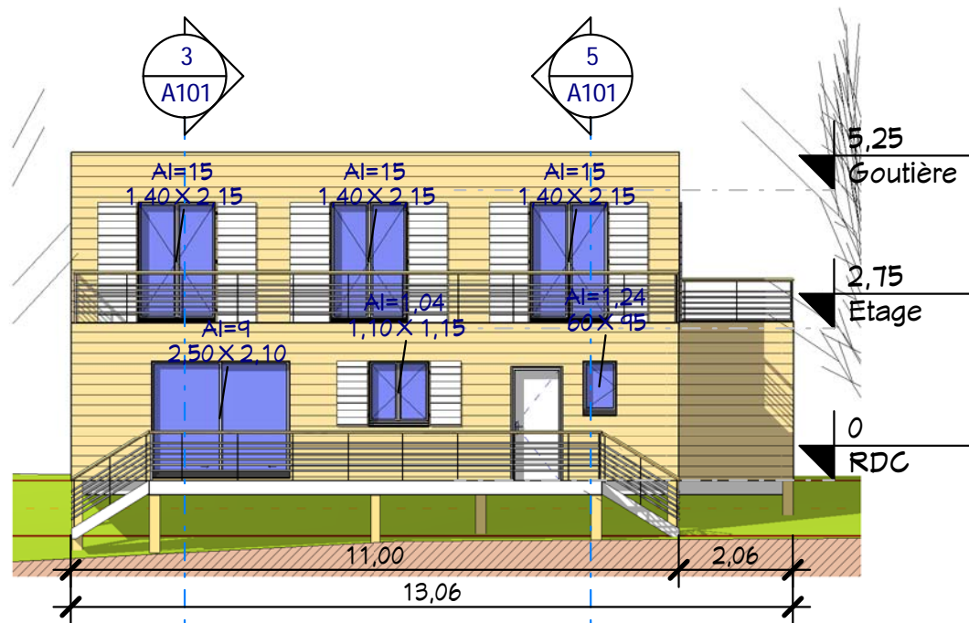
3 Elév. Ouest Ech : 1 : 125
